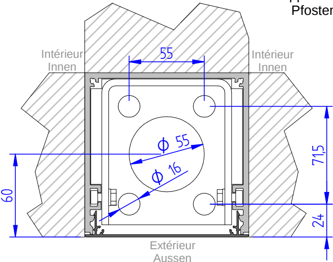
Grondanker Ground anchor Pied fixe à enterrer Grundanker
