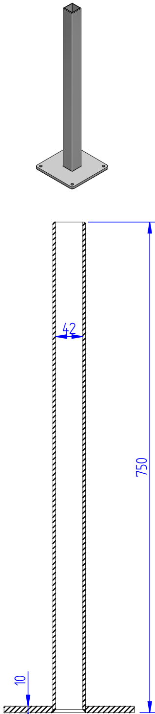
SECTION A-A
